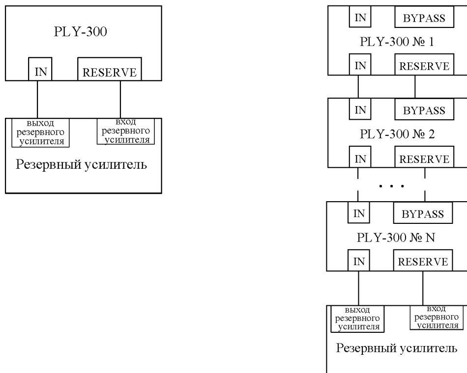
а) схема подключения резервного усилителя при резервировании по схеме «А + В» б) схема подключения резервного усилителя при резервировании по схеме «N + 1»
