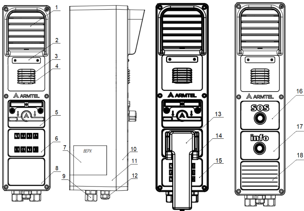
а) ПМЛТ.465311.002, ПМЛТ.465311.002-17
