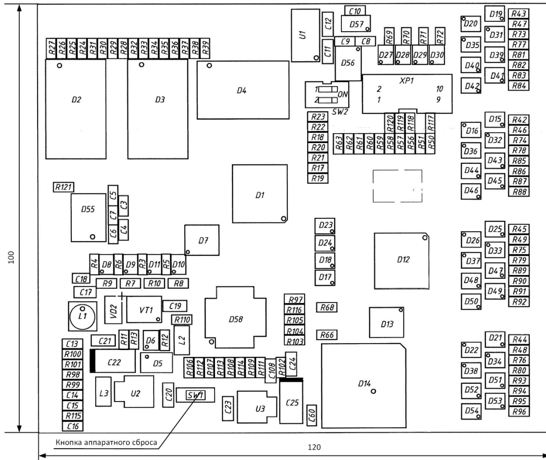
Рисунок 4 – Плата DSP
