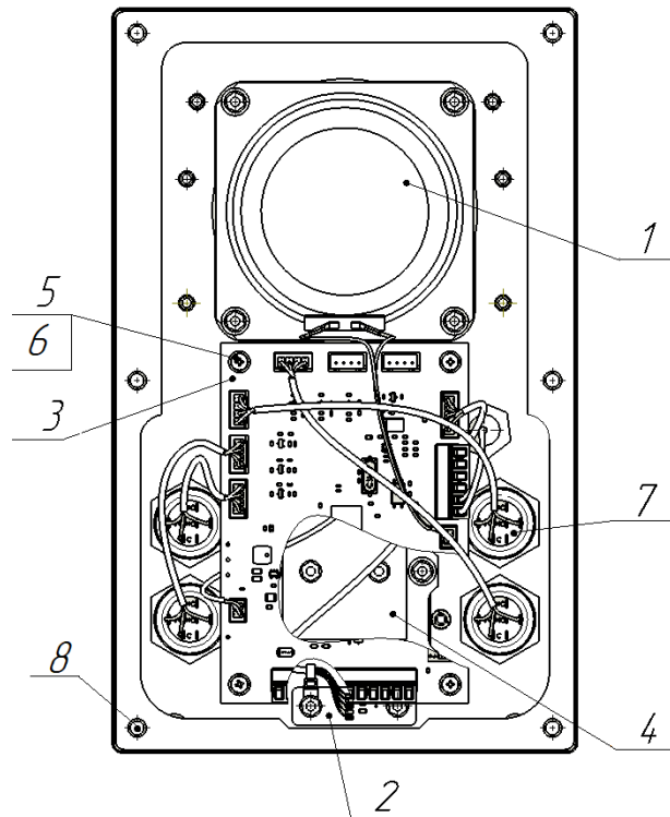
Рисунок 4 – Внутренняя поверхность крышки в CCS-IP2-CR исполнении РМЛТ.465311.021-06 и РМЛТ.465311.021-07
