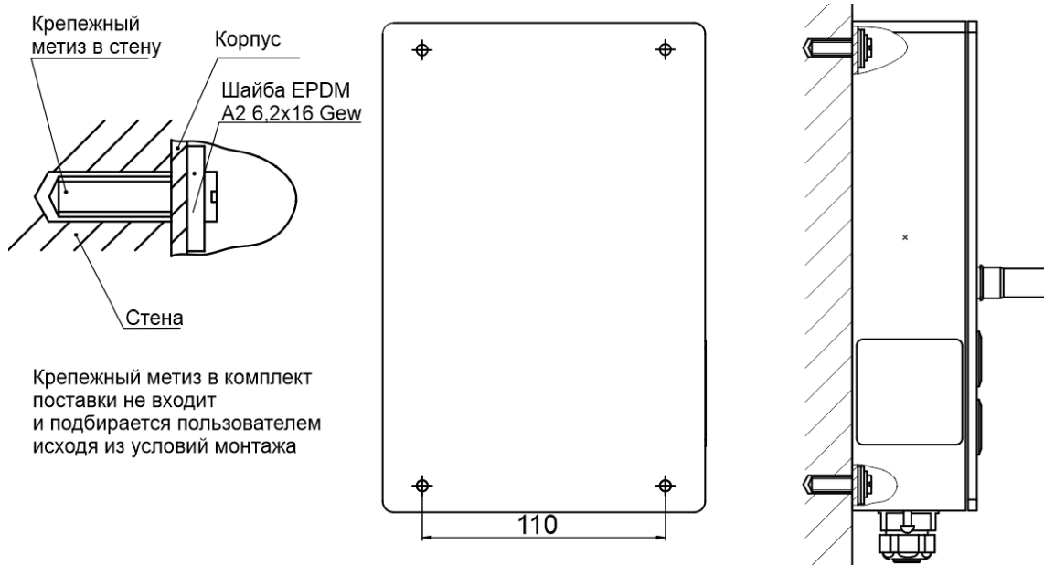
б) установка на стену
