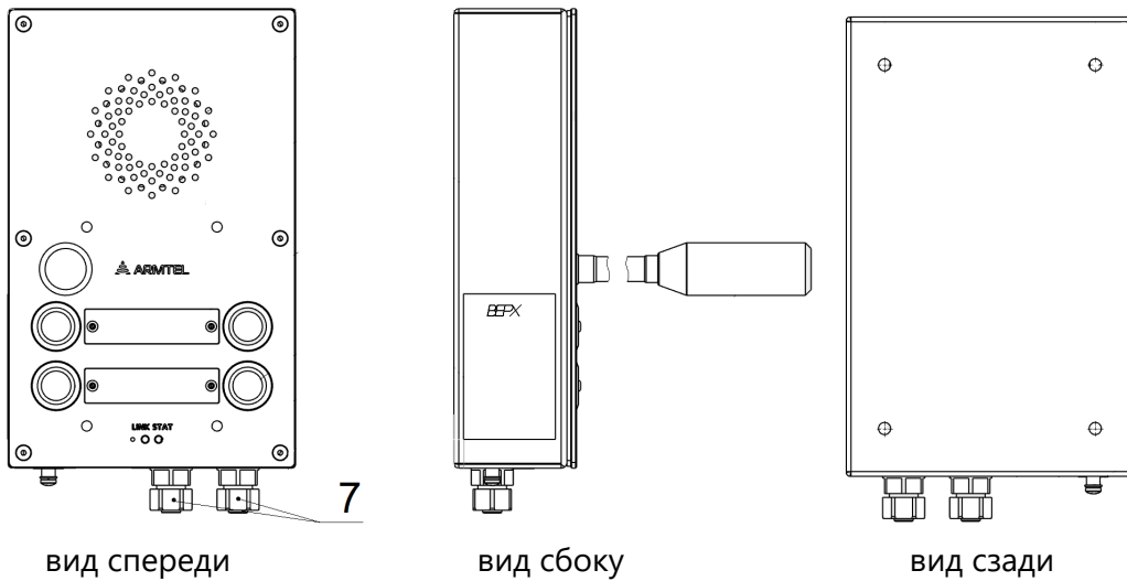
вид спереди вид сбоку вид сзади а) CCS-IP2-CR навесное, исполнения с ПМЛТ.465311.021 по ПМЛТ.465311.021-02
