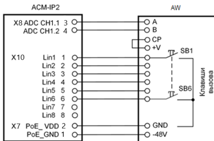
Рисунок А.1 – Подключение аналогового переговорного устройства
